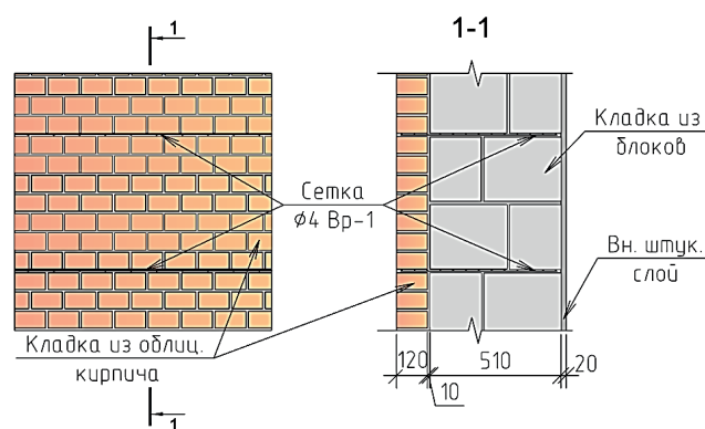
Рис. 1. Схема армирования фрагмента ограждающей конструкции
