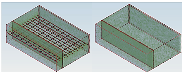
Рис. 2. Расчетные модели фрагмента ограждающей конструкции ( 1000 \times 300 \text{ мм} ) с построением сетки конечных элементов: а) содержащего в своем составе армирующую сетку (модель № 1); б) не содержащего в своем составе армирующую сетку (модель № 2)
